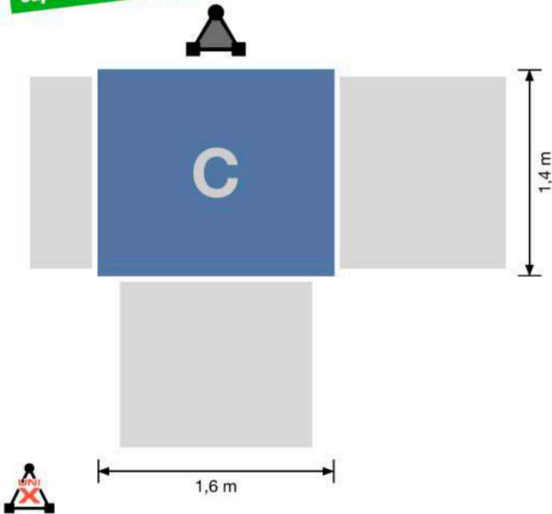
GEDA 500 Z/ZP, plataforma C 2 rampas de carga/1 rampa de descarga
